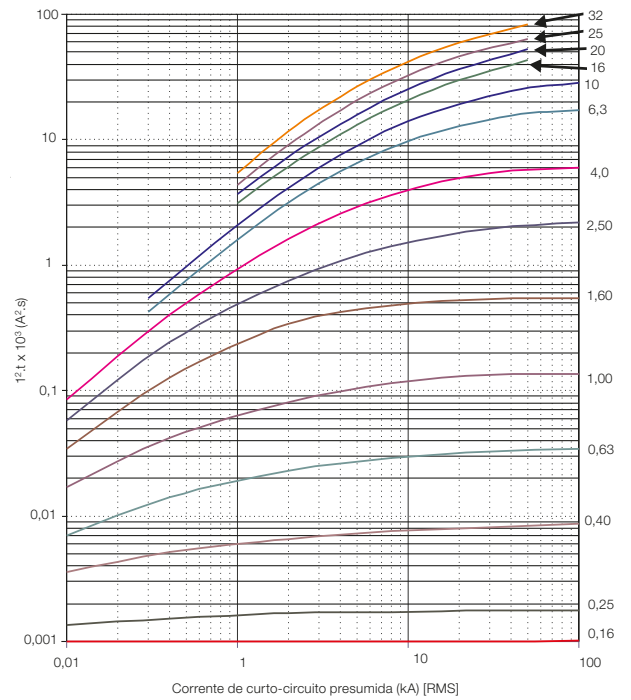
I 2 t em 415 V - MPW40
