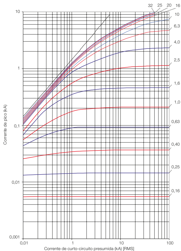
Curva de Limitação de Corrente em Curto-Circuito em 400/415 V - MPW40
