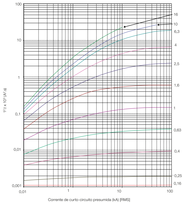
I 2 t em 415 V - MPW12/18
