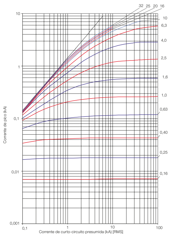
Curva de Limitação de Corrente em Curto-Circuito em 500 V - MPW40
