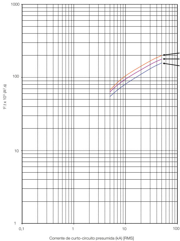
I 2 t em 415 V - MPW80
